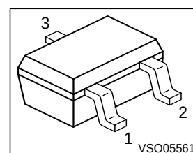
PG-SOT-323
