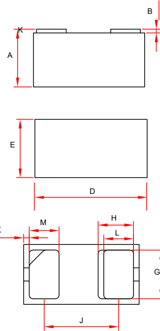
DIMENSIONS
