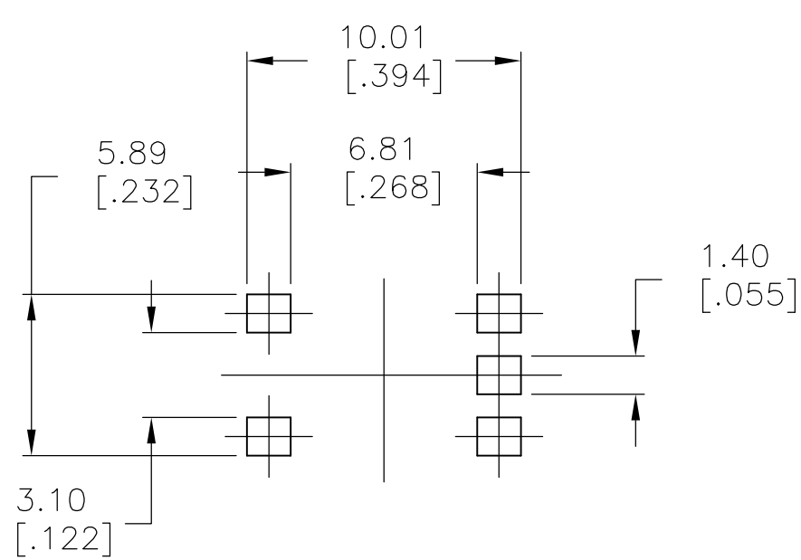
P.C.B. FOOTPRINT
