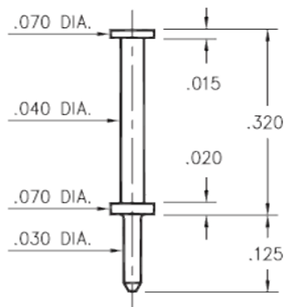
6821-0-00-XX-00-00-08-0 Wire Termination
