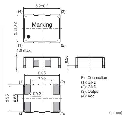
XNCJH, XTCJH 10.0000–52.0000MHz
