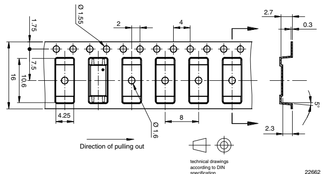
Fig. 21 - Tape Dimensions
