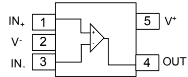
SOT25 / SOT353
