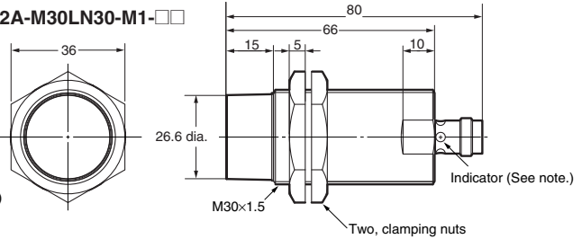
E2A-M30LN30-M1-□□
