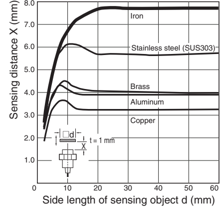
E2A-M18□S08
