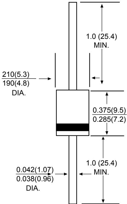
Case Style 1.5KE (DO-201)
