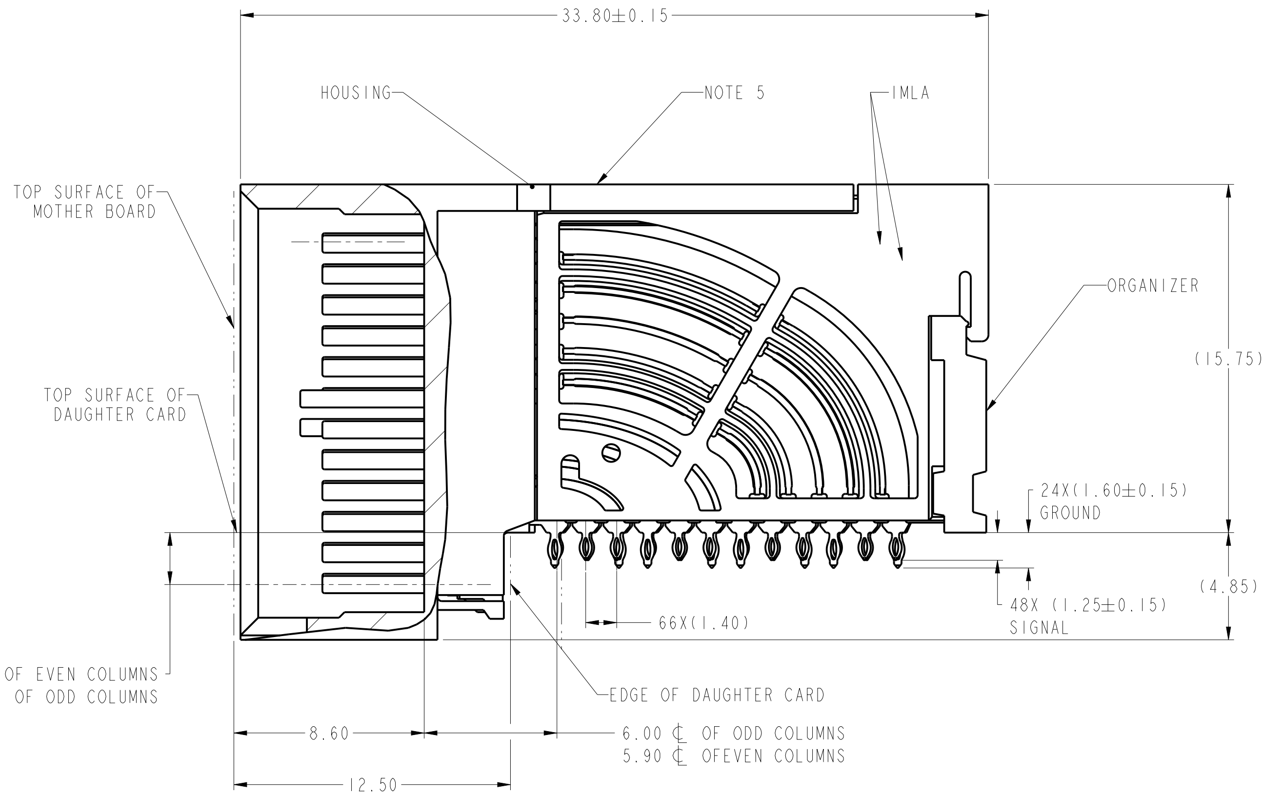
SECTION AA-AA
