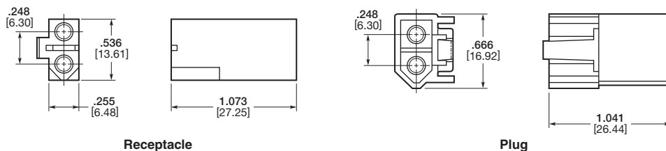
Receptacle
