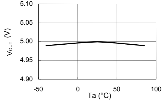
S-817A50A/S-817B50A V_{IN}=7\text{V}, I_{OUT}=10\text{mA}
