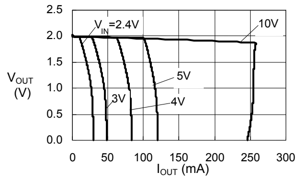
S-817B20A (Ta=25°C)
