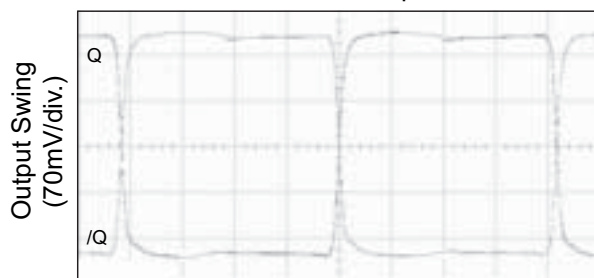
200MHz Output
