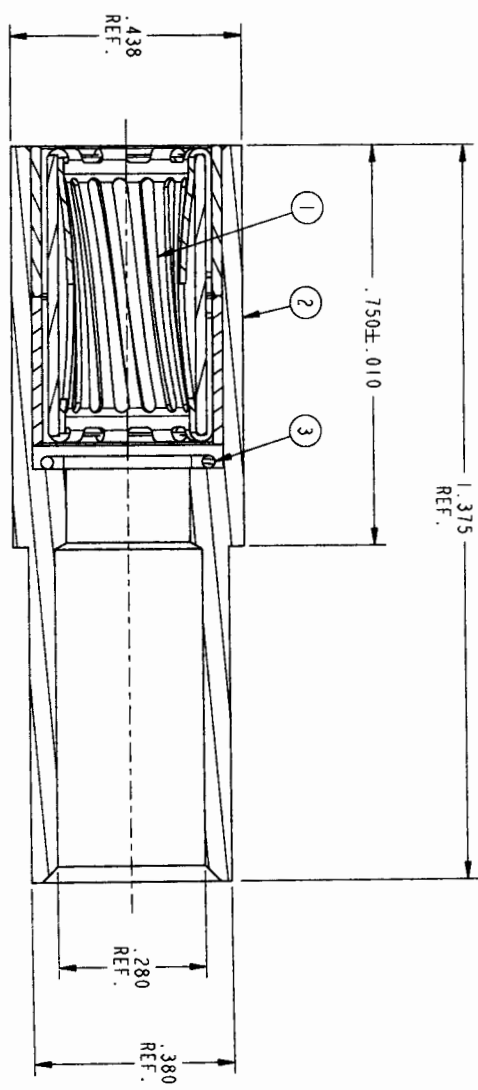
SECTION A-A
