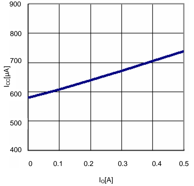
Fig.20 I_o - I_{cc}
