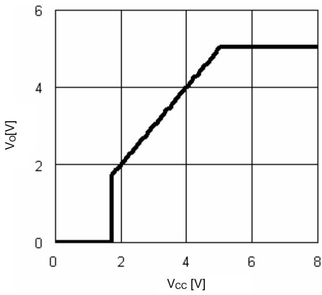
Fig.15 V_{cc}-V_o ( I_o=0mA )
