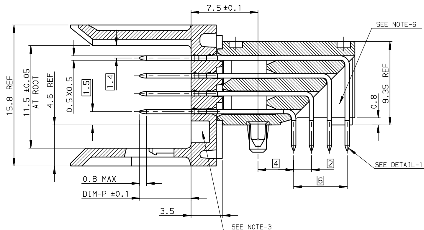
SECTION-A SCALE:4/1
