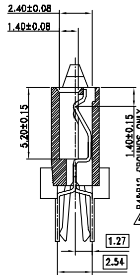
SECTION N-N 2:1
