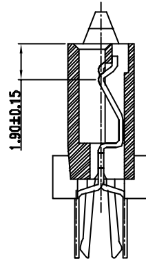
SECTION P-P 2:1
