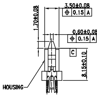
SECTION P-P 2:1
