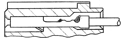
ファスチンファストン嵌合状態 (FASTIN-FASTON MATING STATE)
