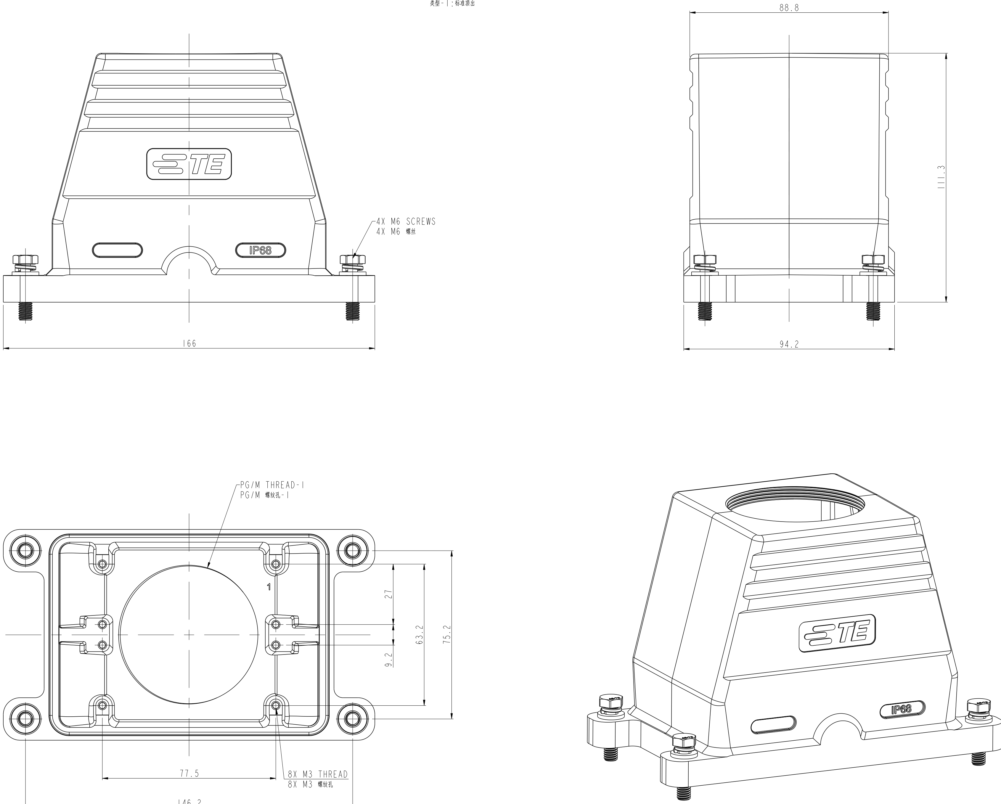
TYPE-1:STANDARD TOP ENTRY 类型-1:标准顶装
