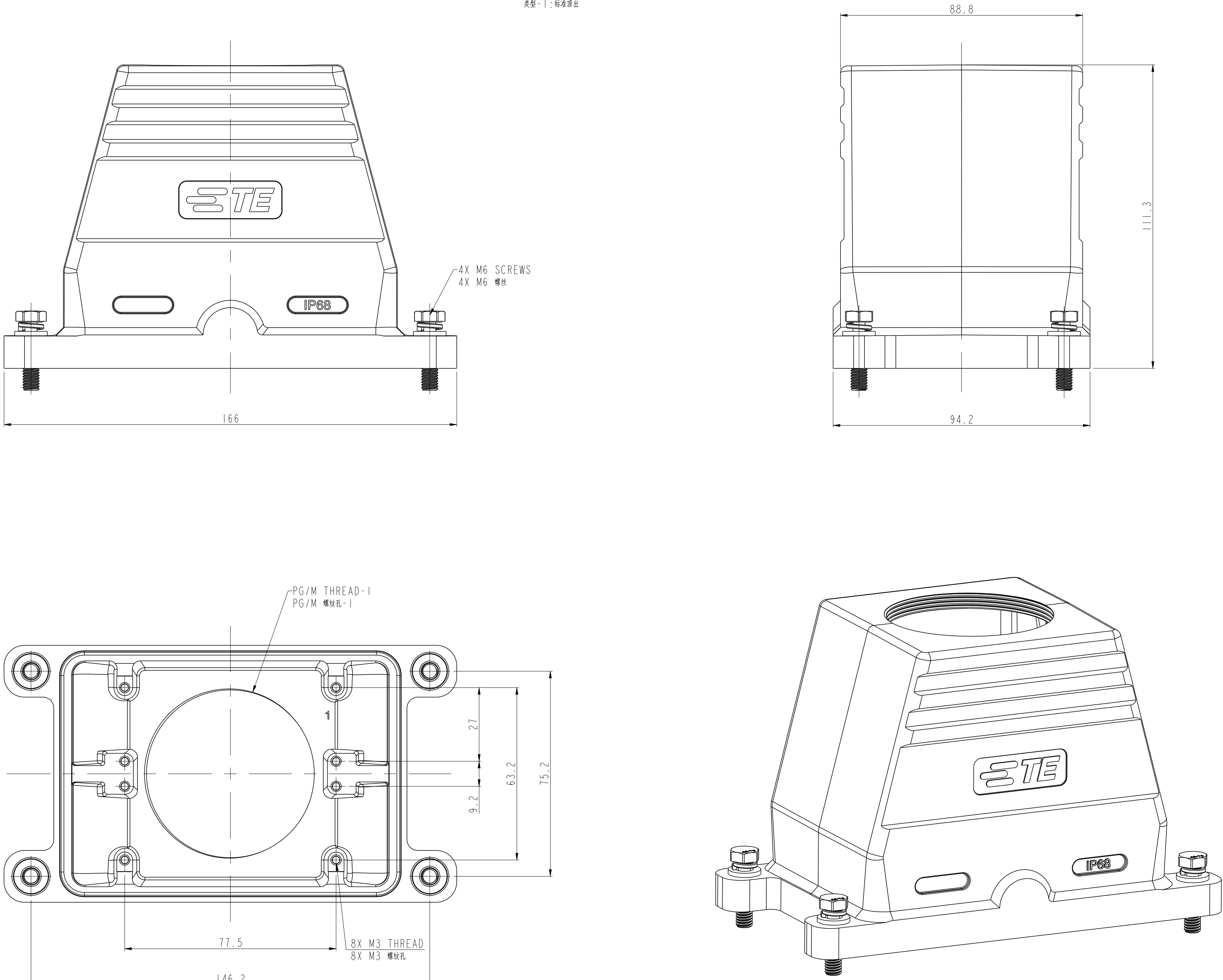
TYPE-1:STANDARD TOP ENTRY 类型-1:标准顶出
