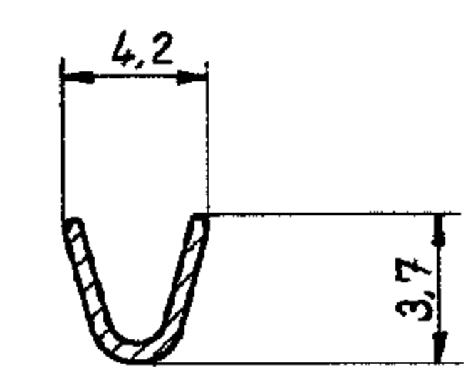
Schnitt A-B
