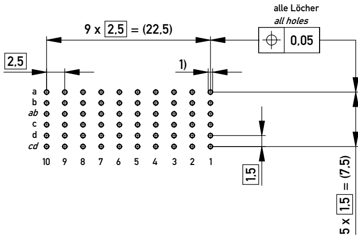
Lochbild für Leiterplatte (Bestückungsseite) board hole pattern (component mounting side)
