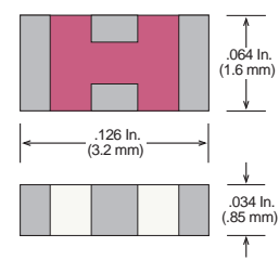
Case 18-2 (EIA 1206 / 3216)
