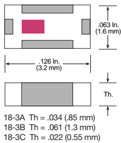
Case 18-3 (EIA 1206 / 3216)
