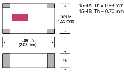
Case 15-4 (EIA 0805 / 2012)
