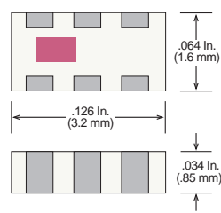
Case 18-1 (EIA 1206 / 3216)
