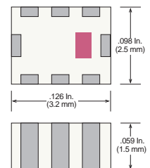
Case 41-2 (EIA 1210 / 3225)
