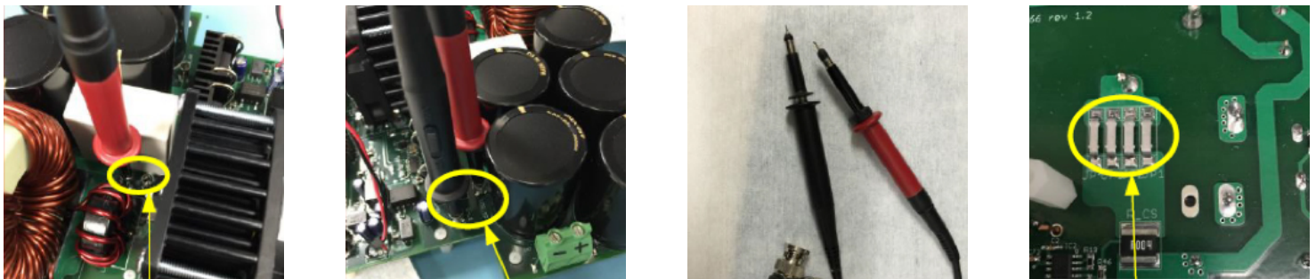
Probing tips: Low side GaN FET V_{GS} and V_{DS}
