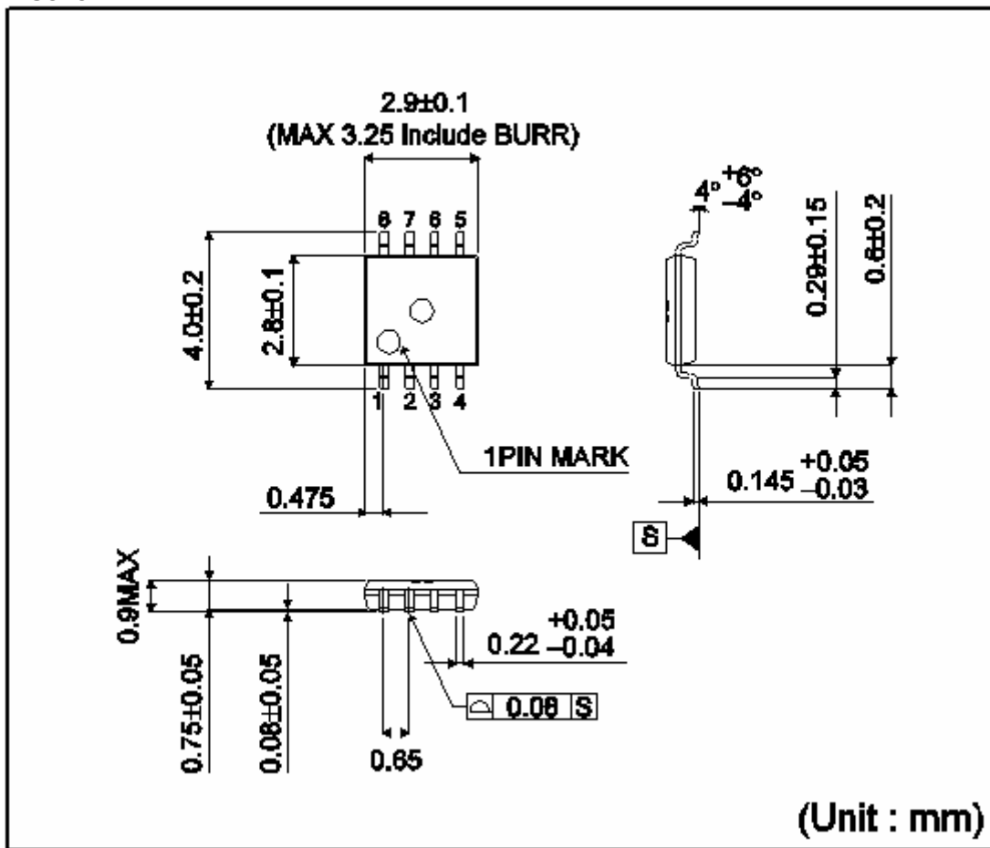
MSOP8
