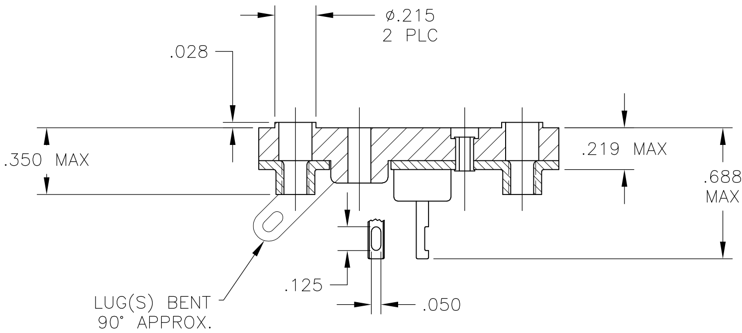
SECTION A-A
