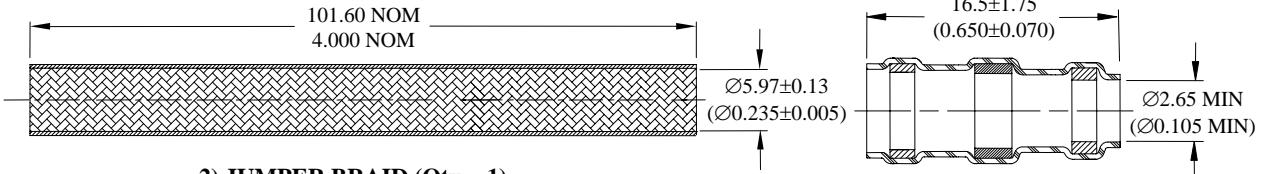
3) SOLDER SLEEVE, Qty.: 2
