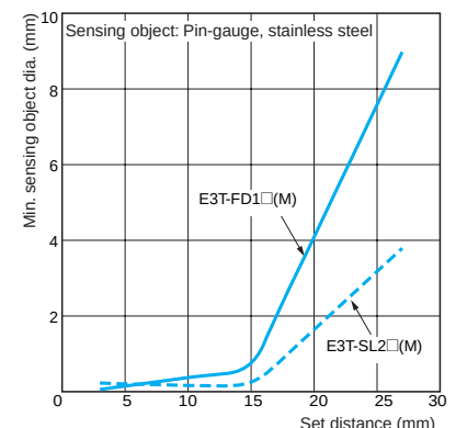
E3T-FD1□(M)/E3T-SL2□(M)
