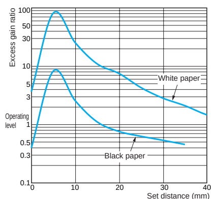
E3T-FD1□(M)
