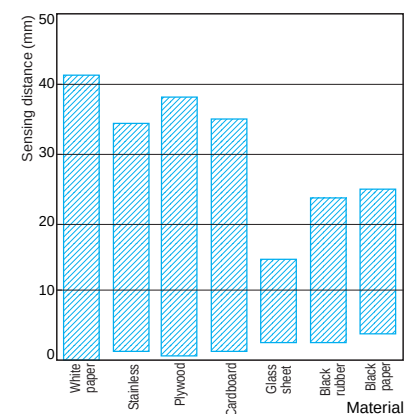
E3T-SL2□(M)
