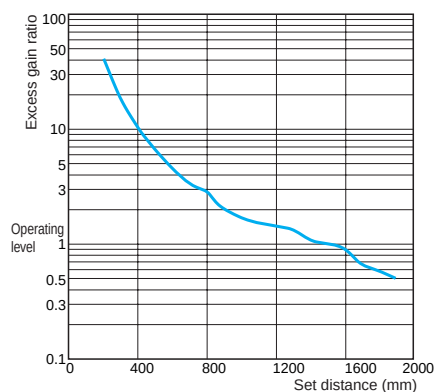
E3T-FD1□(M)
