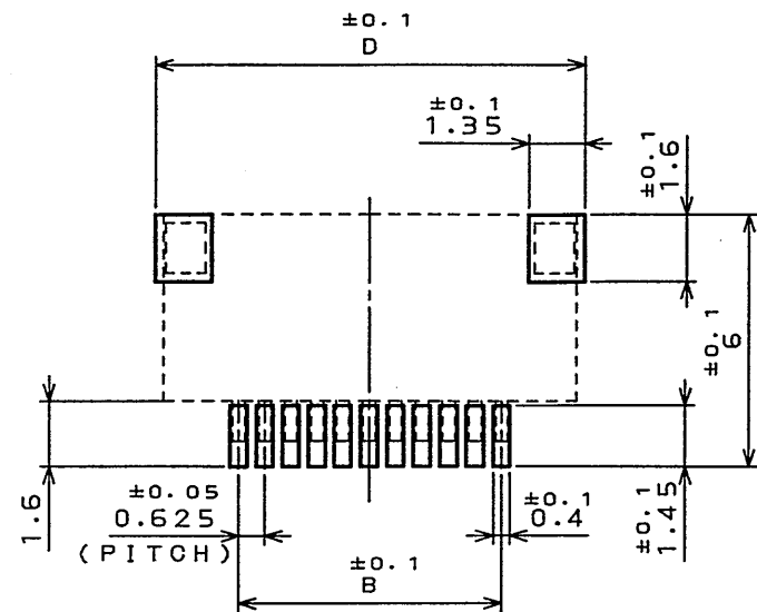
P. C. B. PATTERN DEMENSION(REF.) 基板パターン寸法(参考)
