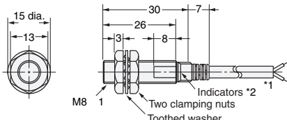
Diagram 5 E2E-X2D□ E2E-X1R5E□/F□
