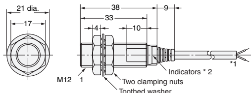
Diagram 9 E2E-X3D□ E2E-X2E□/F□
