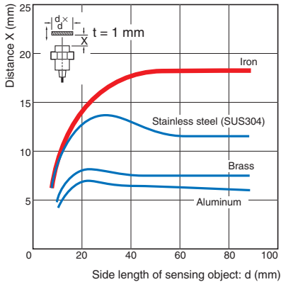
E2E-X18ME/-X18MY/-X18MF
