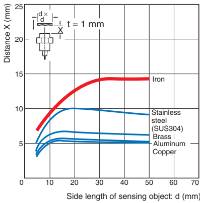
E2E-X2E/-X2Y/-X2F
