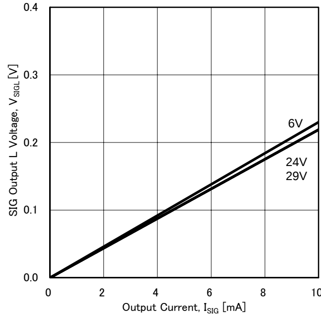
Figure 10. SIG L Voltage (Ta=25°C)
