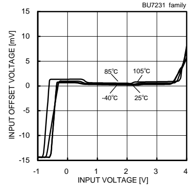
Fig. 59 Input Offset Voltage – Input Voltage (VDD=3[V])
