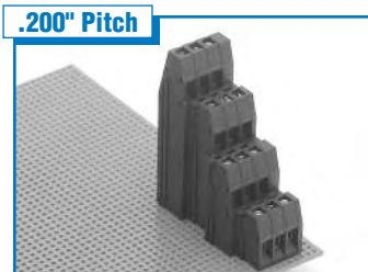
.200" Pitch ESTT 4-tier . . . . . Page 67 24A / 300V
