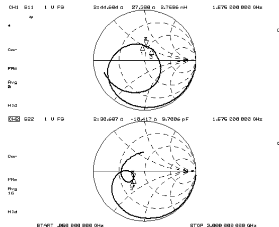
Zin, Zout
