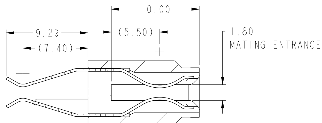
SECTION D-D
