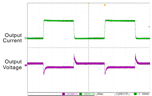
Load Transient I_O=0-1\text{A} , V_O=1.2\text{V} , V_{IN}=5\text{V}
