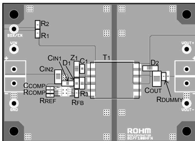
Top Layer
