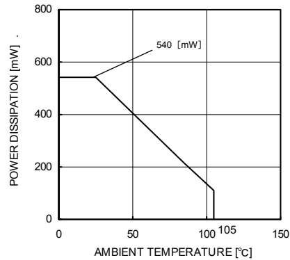
(d) BU7265SG BU7271SG BU7411SG BU7421SG
