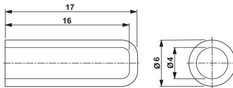
D-SUB filler plug
