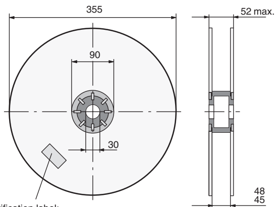
Fig. 18 - Reel
