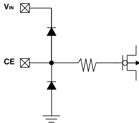
&lt;CE pin&gt;
