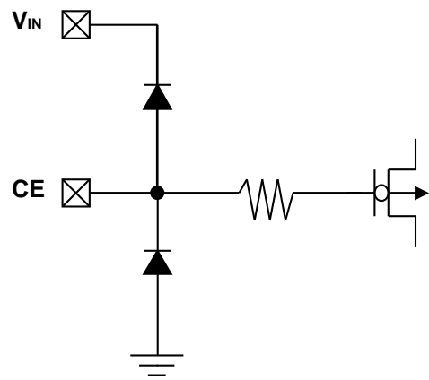
<CE pin>
