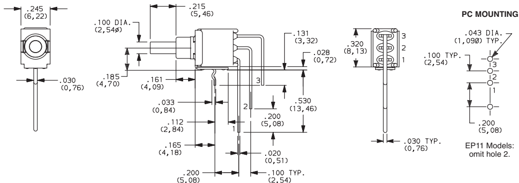
EP12SD1AV3BE SPST
