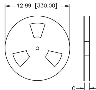
REEL DIMENSIONS
