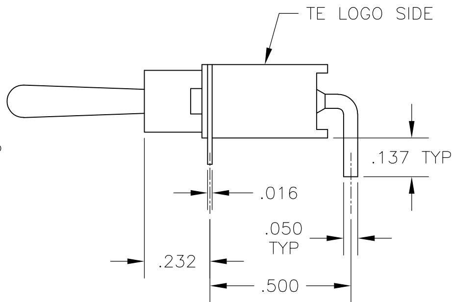
D1 BUSHING
